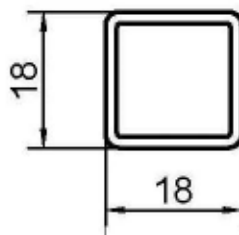
Strebe
